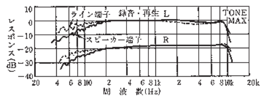
図 63-4 初期のカセットデッキの性能 (Philips EL-3312 の例)
