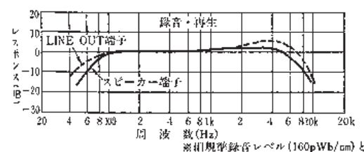
図 63-3 初期のカセット・レコーダーの性能 (Philips EL-3301 の例)
