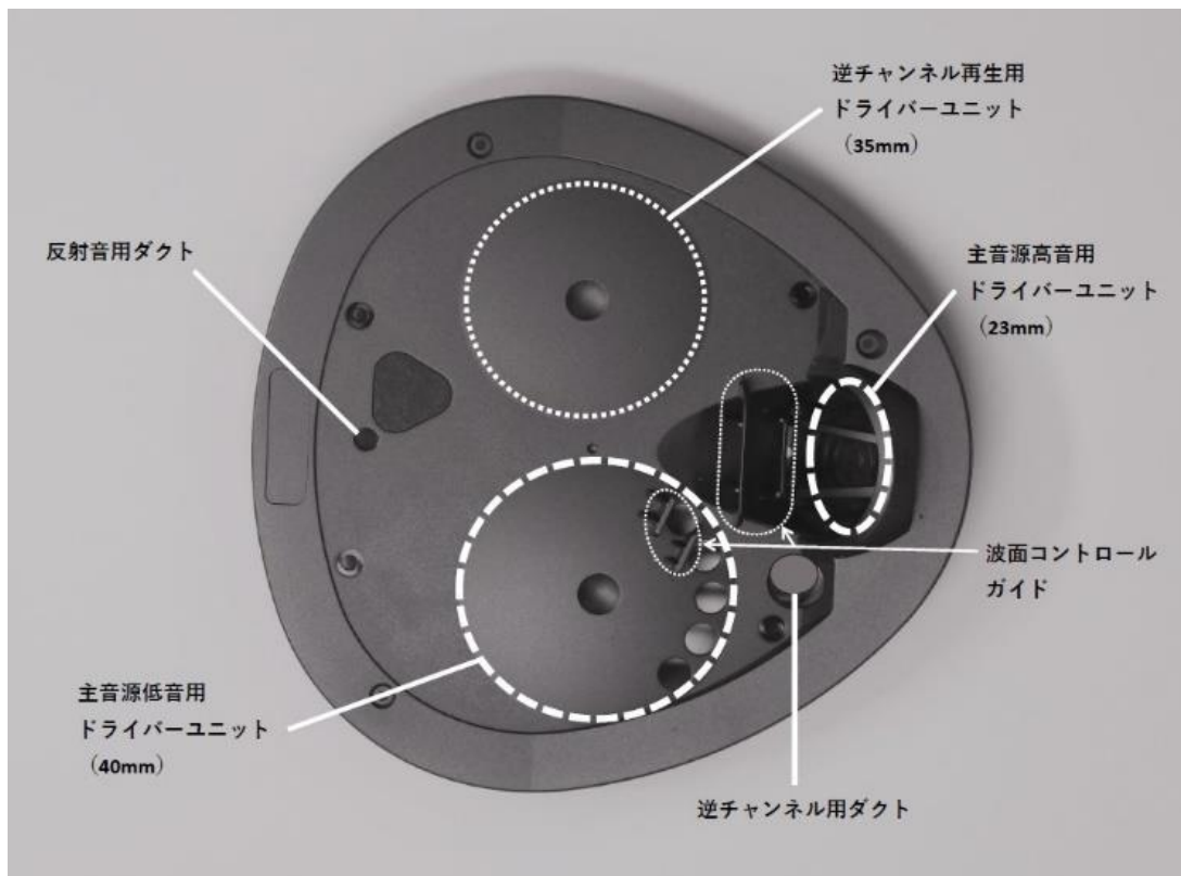
ドライバーユニット配置図
