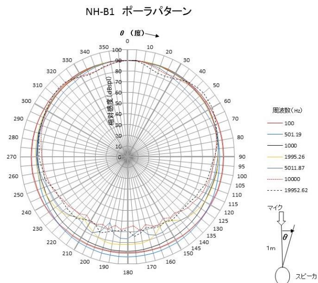
図 たまごスピーカの音圧放射特性
